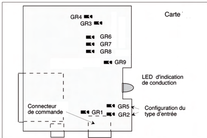
Emplacement des «Grains de café» sur la carte (vue côté soudures)
